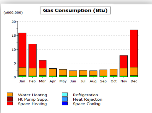
شکل ۳ میزان مصرف گاز به تفکیک ماه های سال و موارد مصرف
