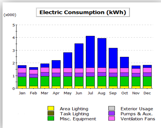
شکل ۲ مصرف انرژی الکتریکی در ساختمان به تفکیک ماه و موارد مصرف
